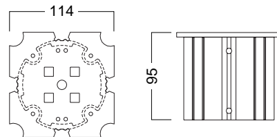
M-Joint A
